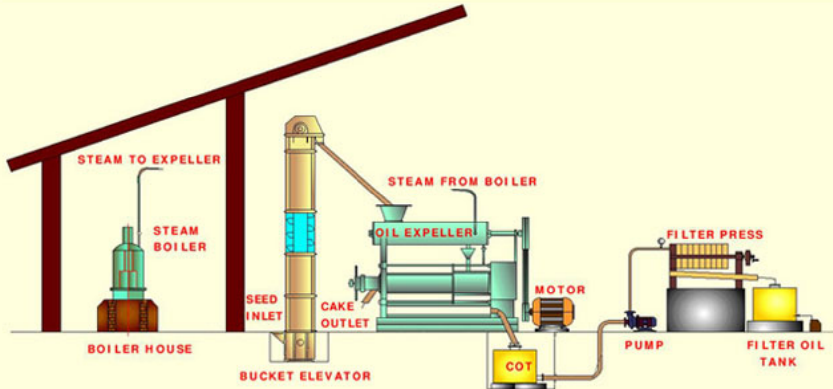
MINI OIL MILL PLANT.
